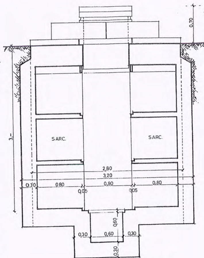
SECCION A-B
