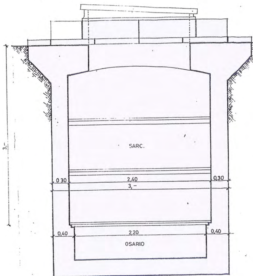
SECCION C-D
