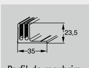
Perfil de recubrim. de cantos aluminio (perfil básico)
