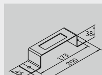
Estribo de fijación
