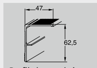
Perfil de recubrim. de cantos aluminio (perfil recubrim.)
