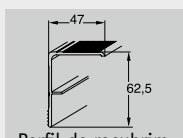
Perfil de recubrim. de cantos aluminio (perfil recubrim.)
