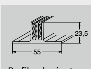
Perfil cubrejuntas de aluminio (perfil básico)
