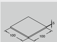
Almohadilla de goma
