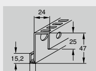
Perfil de conexión de pared de aluminio²
