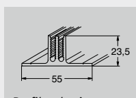
Perfil cubrejuntas de aluminio (perfil básico)
