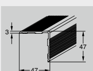
Ángulo de recubrimiento de aluminio
