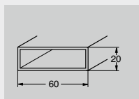
Perfil de subconstrucción de aluminio
