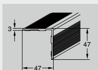
Ángulo de recubrimiento de aluminio
