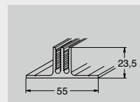
Perfil cubrej. aluminio (perfil básico)
