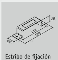
Estribo de fijación
