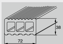
Rastrel de subconstrucción bz¹
