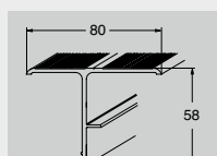
Perfil cubrej. aluminio (perfil recubrim.)
