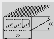
Rastrel de subconstrucción bz¹
