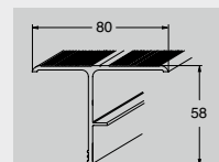
Perfil cubrej. aluminio (perfil recburim.)
