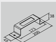
Estribo de fijación
