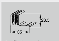
Perfil de recubrim. de cantos aluminio (perfil básico)
