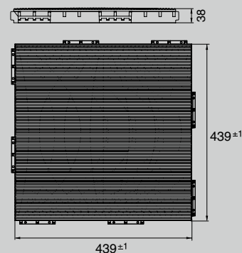
Cassette para terrazas terraza
