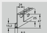
Perfil de conexión de pared de aluminio²
