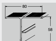
Perfil cubrej. aluminio (perfil recubrim.)
