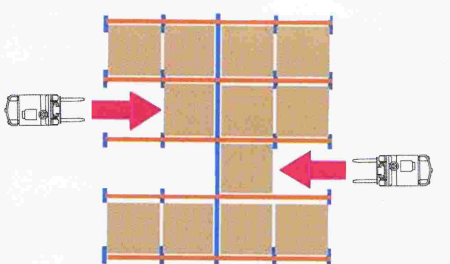
Estantería Drive-In de entrada doble
