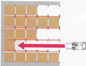
Estantería Drive-In de entrada simple
