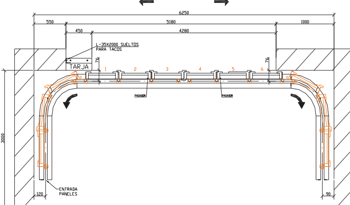
DETALLE HOJAS Y GUIA INFERIOR
