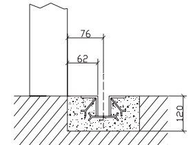
DETALLE GUIA INFERIOR
