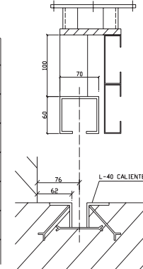
DETALLE GUIAS SUPERIOR E INFERIOR
