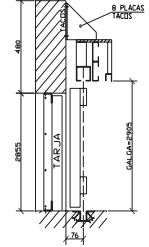
DETALLE GUIA INFERIOR
