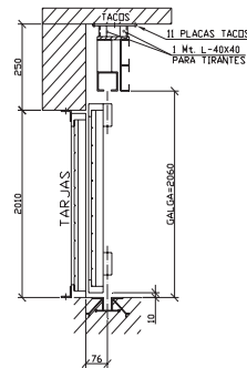
DETALLE GUIAS SUPERIOR E INFERIOR
