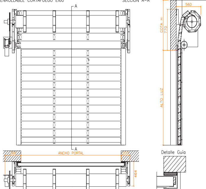
ENROLLABLE CORTAFUEGO E160
