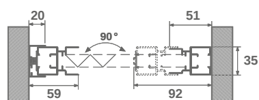
SECCIÓN HORIZONTAL 3 HOJAS
