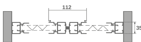
SECCIÓN HORIZONTAL 4 HOJAS
