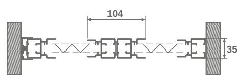
SECCIÓN HORIZONTAL 2 HOJAS A SEGUIR
