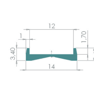
CALZO MARCO Perimetral
