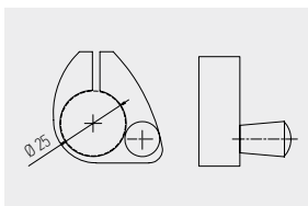
9018 BATENTE EM AÇO INOX PARA SISTEMA DESLIZANTE (DRT/ ESQ INDICAR NO PEDIDO)
