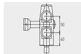
7402 SUPORTE BANDEIRA COM FIXAÇÃO LATERAL E RECEPTOR DE PIVOT EM AÇO INOX PARA REF.ª 7101 VIDRO: 10mm
