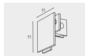
522 UNIÃO DE 2 A 3 VIDROS COM BATENTE E CONTRAVENTAMENTO VIDRO: 10mm ENTALHE: 4 MX
