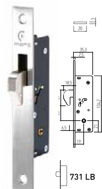
731 LG FECHADURA C/ CILINDRO CRUZ min. 20 un.
