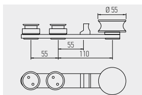
9001 ROLDANA COM SUPORTE EM AÇO INOX PARA SISTEMA DESLIZANTE COM TRAVAMENTO VARÃO
