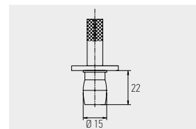
7451 PIVOT EM AÇO INOX PARA PEÇA REF.ª 7101
