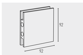
2613 TESTA SEM BATENTE PARA VIDRO DA FECHADURA REF.ª 613 VIDRO: 10mm ENTALHE: M612
