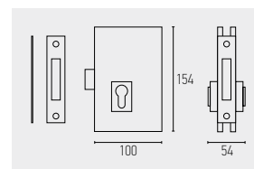
642 FECHADURA EM AÇO INOX PARA PORTA INDIVIDUAL SEM MULETA VIDRO: 10mm EN 12209
