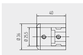
9015 TOPO DE FIXAÇÃO DE VARÃO À PAREDE EM AÇO INOX
