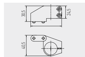
9004 BATENTE EM AÇO INOX PARA SISTEMA DESLIZANTE (DRT/ ESQ INDICAR NO PEDIDO)
