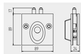
613 FECHADURA UNIVERSAL COMPLETA VIDRO: 10mm ENTALHE: M612 EN 12209
