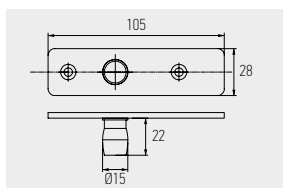
7452 BASE COM PIVOT EM AÇO INOX PARA PEÇA REF.ª 7101 VIDRO: 10mm
