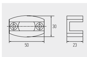
9005 GUIA EM AÇO INOX PARA SISTEMA DESLIZANTE (VIDRO DE 8 A 12 mm)
