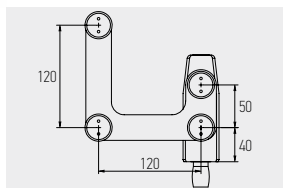
7401 FIXAÇÃO DE BANDEIRA E MONTRA E RECEPTORA DE PIVOT EM AÇO INOX VIDRO: 10mm
