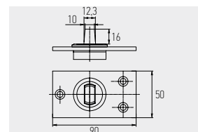
7463 EIXO ROTATIVO EM AÇO INOX PARA PEÇA REF.ª 7132 VIDRO: 10mm
