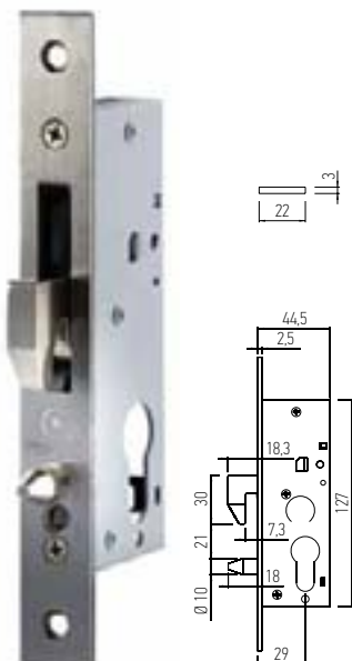
732 FECHADURA PICO-LORO min. 20 un.
