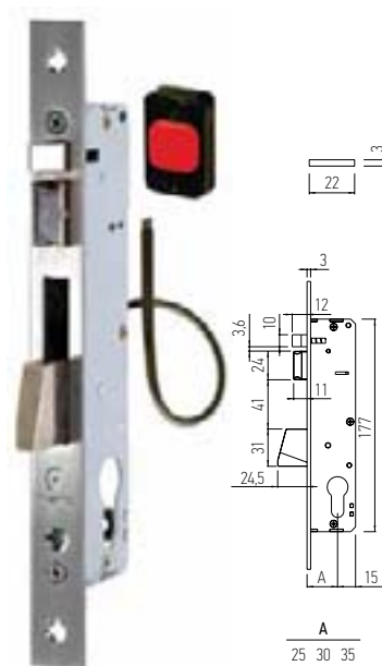
733 ⚡ FECHADURA PRUMO (ELÉCTRICA) min. 20 un.
