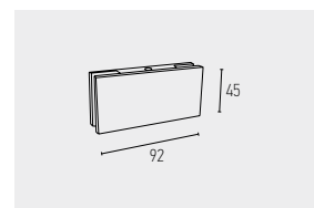
5001 PEÇA DE FIXAÇÃO CENTRAL DE 1 OU 2 VIDROS VIDRO: 10mm ENTALHE: 2 MX
