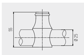
9017 BATENTE EM AÇO INOX PARA SISTEMA DESLIZANTE
