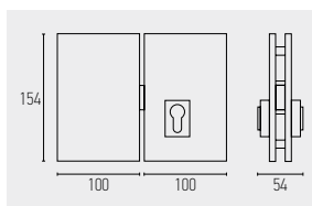
641 FECHADURA EM AÇO INOX PARA PORTA DUPLA SEM MULETA VIDRO: 10mm EN 12209
