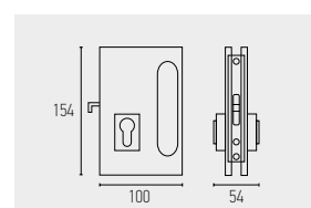
9027 FECHADURA EM AÇO INOX PARA PORTA DE CORRER SIMPLES VIDRO: 10mm EN 12209
