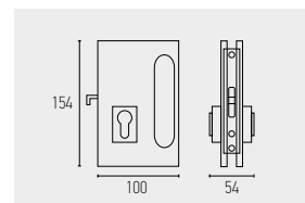
9027 FECHADURA EM INOX PARA PORTA DE CORRER SIMPLES VIDRO: 10mm EN 12209
