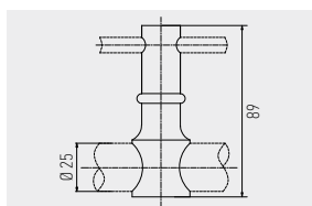
9016 BATENTE EM AÇO INOX PARA SISTEMA DESLIZANTE COM TRAVAMENTO NA ROLDANA
