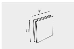
514 UNIÃO DE 2 VIDROS COM 4 FUROS VIDRO: 10mm ENTALHE: 4 MX
