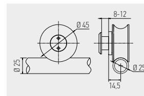
9012 FIXADOR VIDRO/VARÃO Ø25 EM AÇO INOX
