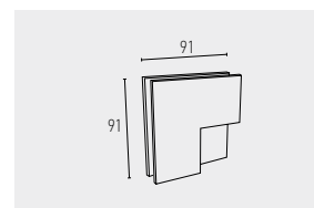
519 UNIÃO DE 2 A 3 VIDROS COM BATENTE VIDRO: 10mm ENTALHE: 3 MX
