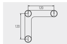
7521 FIXAÇÃO DE BANDEIRA E MONTRA EM AÇO INOX VIDRO: 10mm
