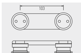
7572 UNIÃO DE 2 VIDROS EM AÇO INOX VIDRO: 10mm
