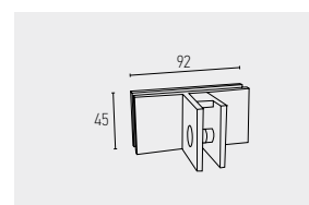
533 FIXAÇÃO CENTRAL COM CONTRAVENTAMENTO E SEM BATENTE VIDRO: 10mm ENTALHE: 3 MX
