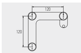
7519 FIXAÇÃO DE BANDEIRA E MONTRA EM AÇO INOX COM BATENTE PARA PORTA VIDRO: 10mm
