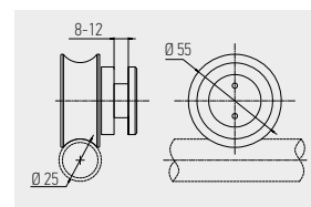
9009 ROLDANA EM AÇO INOX PARA SISTEMA DESLIZANTE
