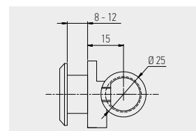
9013 FIXADOR VIDRO/VARÃO Ø25 EM AÇO INOX
