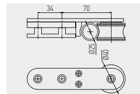
9019 ROLDANA COM SUPORTE EM AÇO INOX PARA SISTEMA DESLIZANTE
