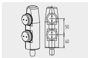
7403 SUPORTE BANDEIRA E RECEPTOR DE PIVOT EM AÇO INOX PARA PEÇA REF.ª 7101 VIDRO: 10mm
