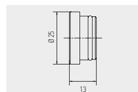
9007 TOPO EM AÇO INOX PARA VARÃO Ø25
