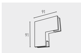
521 UNIÃO DE 2 A 3 VIDROS SEM BATENTE VIDRO: 10mm ENTALHE: 3 MX
