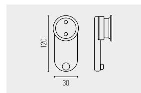
7049 BATENTE EM AÇO INOX PARA PORTA COM BANDEIRA VIDRO: 10mm
