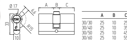
E500 CILINDRO ALTA SEGURANÇA MARQUES min. 10 un.
