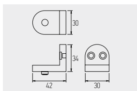
7687 BATENTE EM AÇO INOX PARA PORTA SIMPLES
