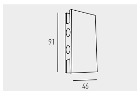
605 FÊMEA DA FECHADURA REF. a 613 SEM BATENTE VIDRO: 10mm ENTALHE: M2X
