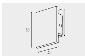
5049 PEÇA DE FIXAÇÃO À BANDEIRA COM BATENTE (E/D) VIDRO: 10mm ENTALHE: MX
