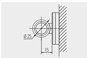
9011 FIXADOR PAREDE/VARÃO Ø25 EM AÇO INOX
