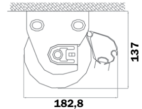
Instalación en el techo (en mm.)
