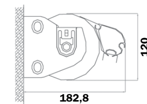
Instalación en la pared (en mm.)
