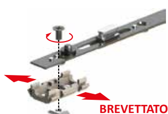
Ejemplo de fijación con adaptador de expansión
