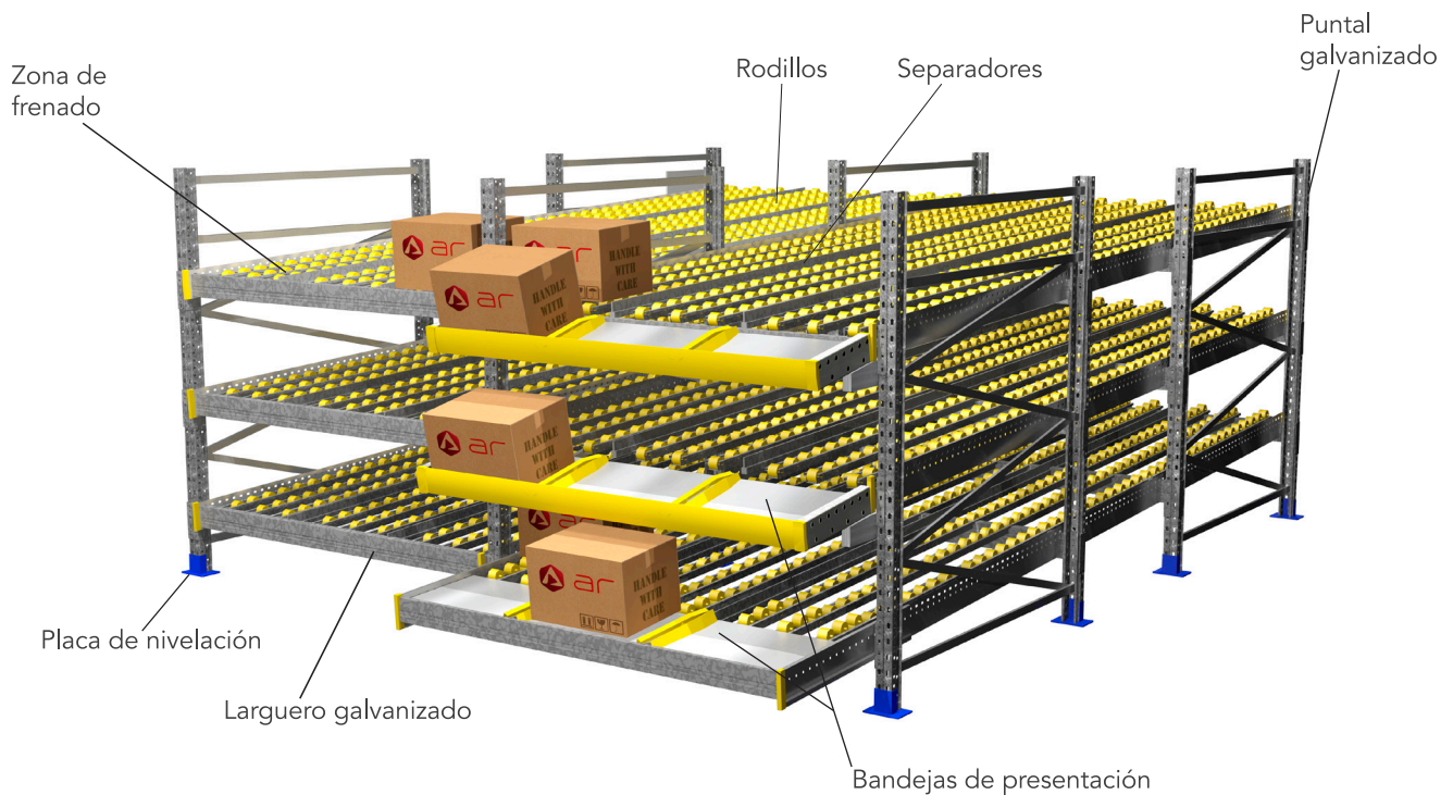
Ejemplo de estantería paletización
