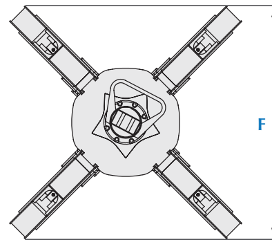
Dimensiones exteriores 4 garras
