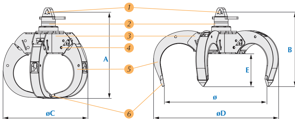
Dimensiones exteriores 4 garras
