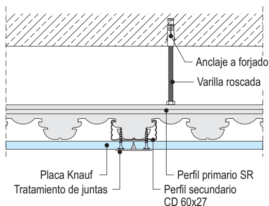
D114-C4 Tratamiento de Junta Transversal Cantos Biselados
