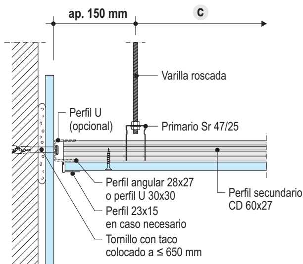
D114-A3 Encuentro con Muro: Junta Vista
