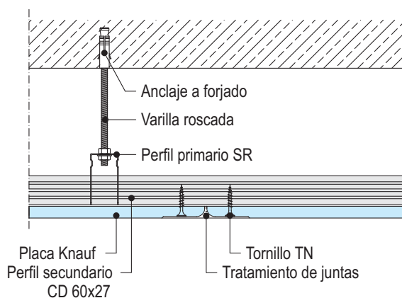
D114-B4 Detalle de Junta Longitudinal
