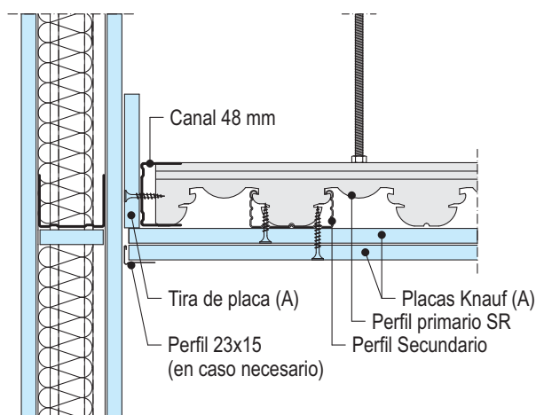
D114-D5 Encuentro con Tabique para Resistencia al Fuego EI 30
