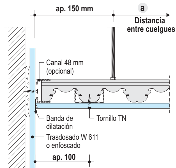
D114-D3 Encuentro con Muro
