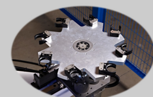
Cambio de herramienta revolver
