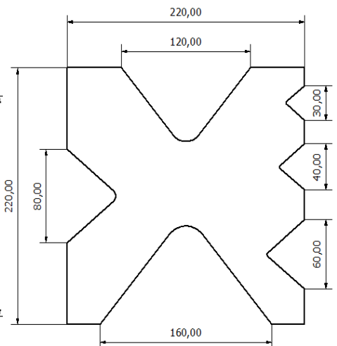
Matriz 320Tn
