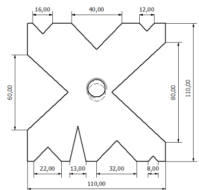
Matriz 160Tn
