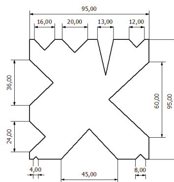
Matriz 125Tn
