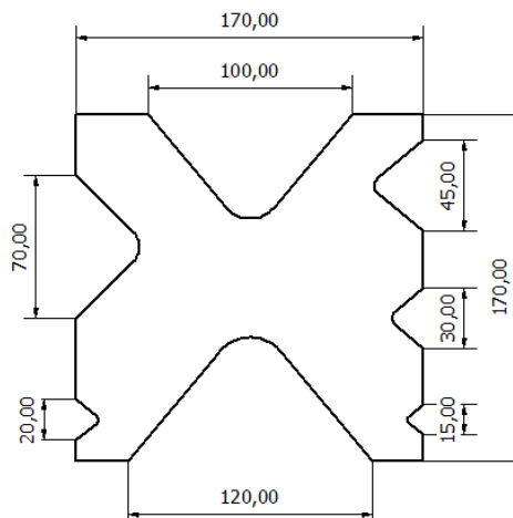
Matriz 250Tn
