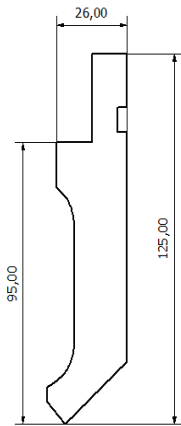
Punzón 50-125Tn
