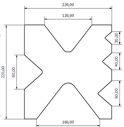
Matriz 160Tn
