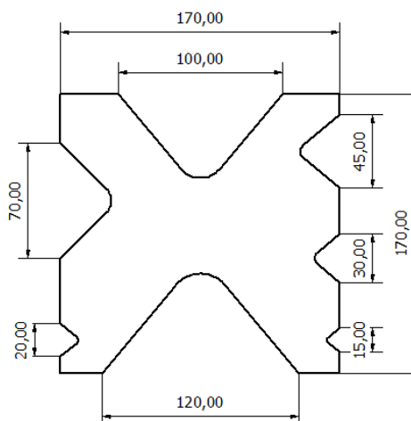
Matriz 250Tn
