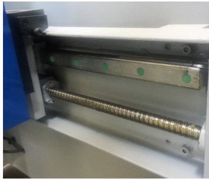
2.- Husillo de bolas y patín guía
