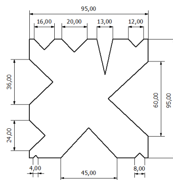
Matriz 125Tn
