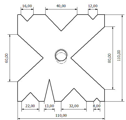
Matriz 160Tn
