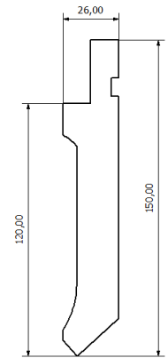
Punzón de 125-260Tn
