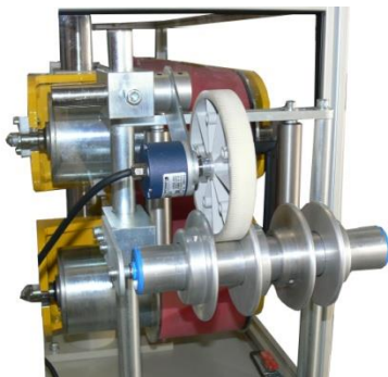
Dispositivo de medición por encoder
