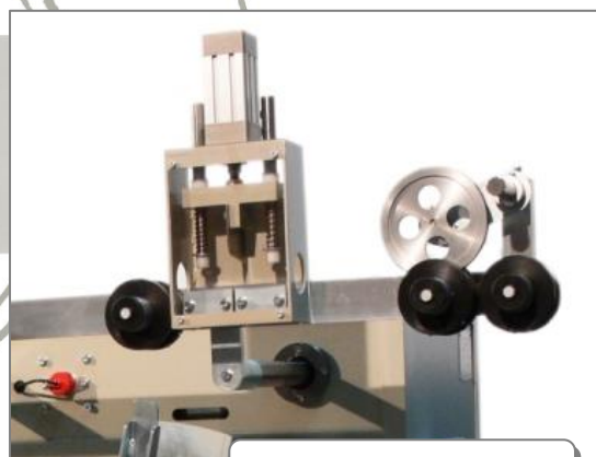
Cortadora neumática
