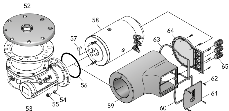
MOTORREDUCTOR 1700W
