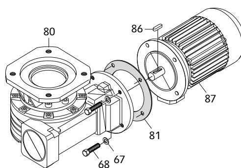
MOTORIDUTTORE 3000 TR
