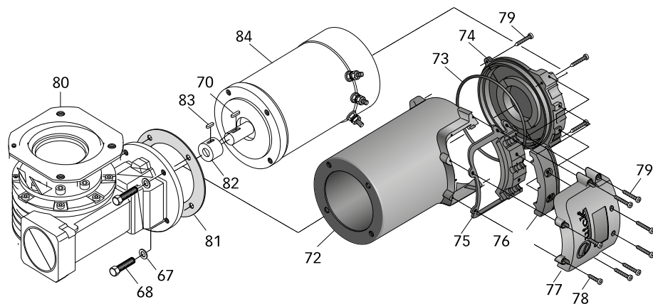
MOTORREDUCTOR 3000W
