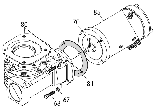
MOTORREDUCTOR 3000W
