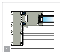
Puerta corredera elevadora en PVC con hoja lateral fija
