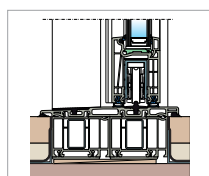
solera ancha con doble ampliación empotrada
