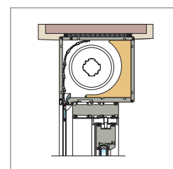
conexión con cajon Mini
