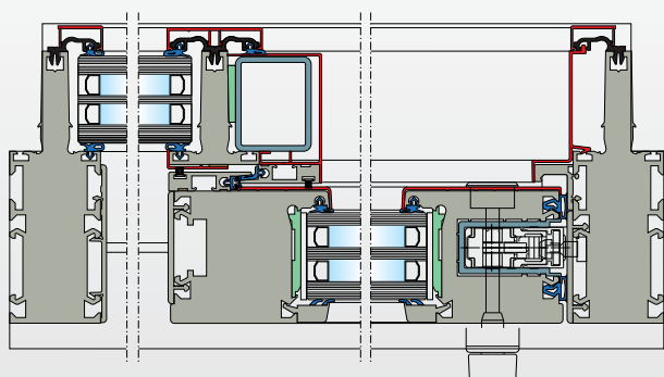
sección horizontal puerta corredera elevadora Vista de PVC-aluminio (KAB)
