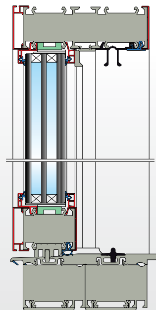
sección vertical puerta corredera elevadora de aluminio
