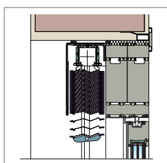
conexión con Raffstore con chapa de revestimiento
