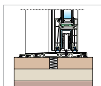
guía corredera sobre suelo acabado
