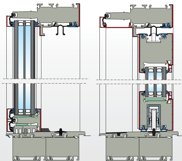
sección vertical puerta corredera elevadora Vista con revestimiento de aluminio en ambos lados
