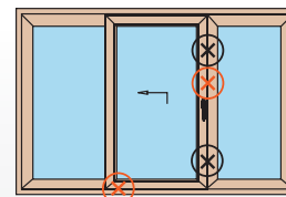
anchura máxima: 5.960 mm altura máxima: 2.800 mm
