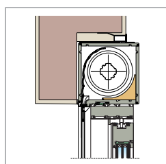
conexión con cajon mini
