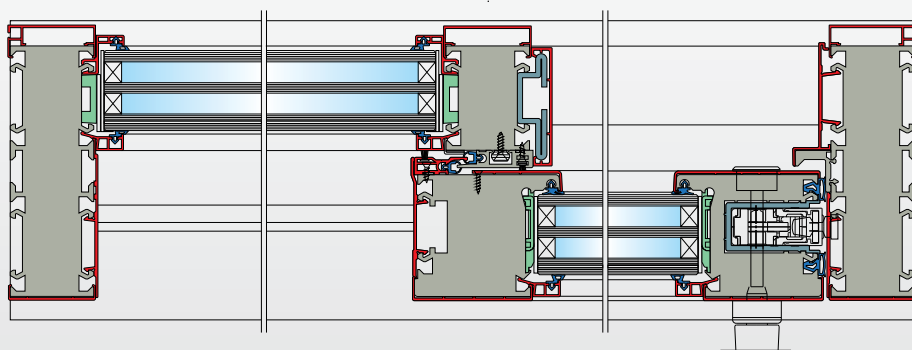
sección horizontal puerta corredera elevadora de aluminio
