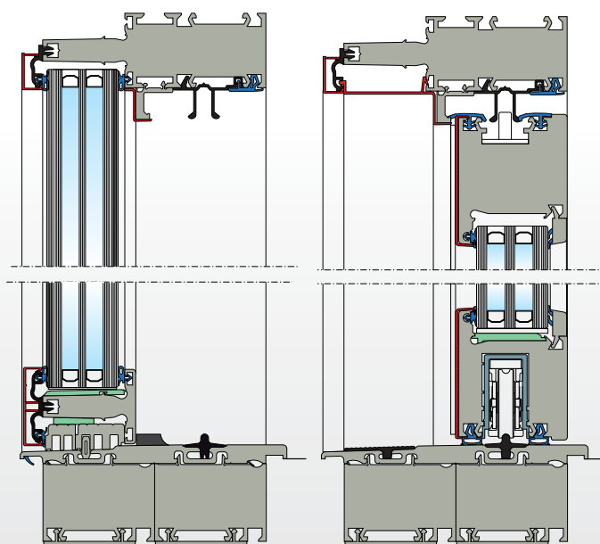
sección vertical puerta corredera elevadora Vista de PVC-aluminio (KAB)
