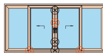
anchura máxima: 5.960 mm altura máxima: 2.800 mm
