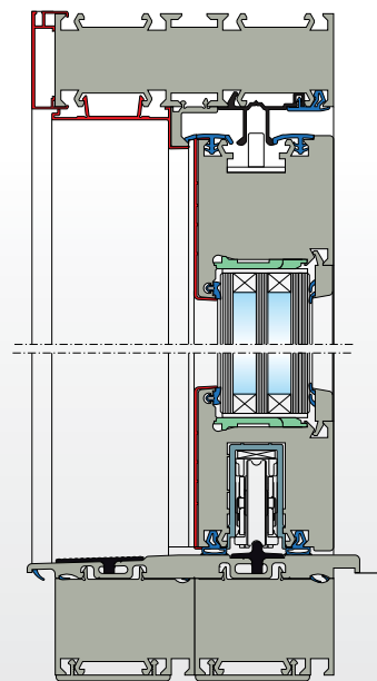
sección vertical puerta corredera elevadora en PVC-aluminio
