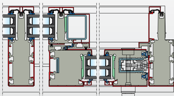
sección horizontal frontal acristalado Vista con puerta corredera elevadora integrada
