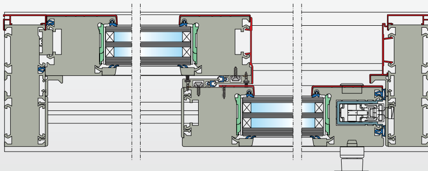
sección horizontal puerta corredera elevadora en PVC-aluminio
