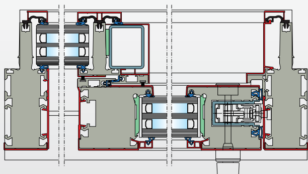
sección horizontal puerta corredera elevadora Vista con revestimiento de aluminio en ambos lados
