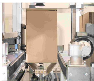
Sistema de plegado de solapas inferiores y aplicación de cola altamente eficiente.
