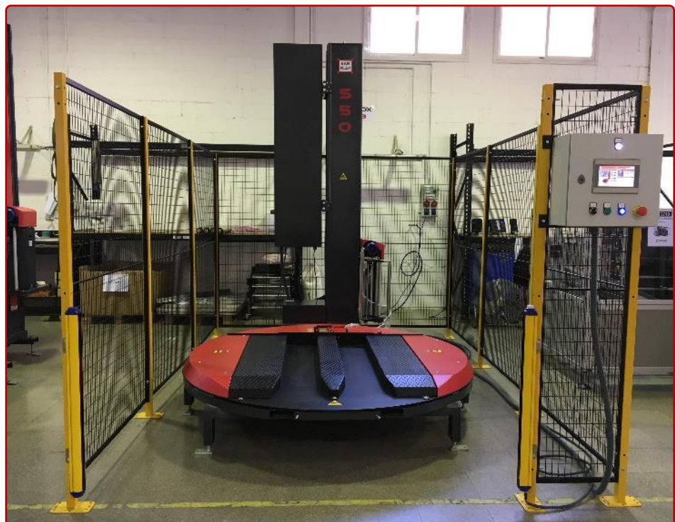
Plataforma con sistema 3ALL incorporado y alzas para envolver carga y palet
