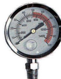
Manómetro de glicerina GYM Metalico 1/4 - 100 bar
