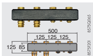
Colector para 2 o 3 circuitos - Bulto EA 140
