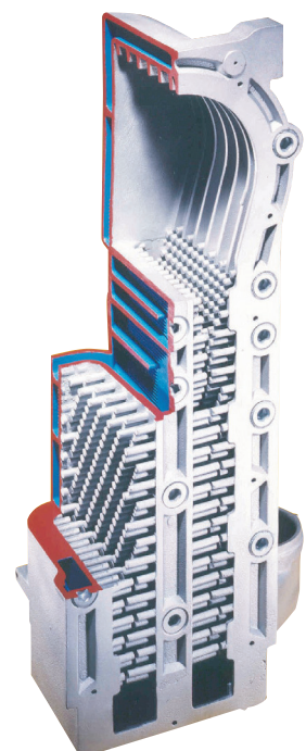
Detalles cuerpo de calefacción de fundición aluminio/silicio
