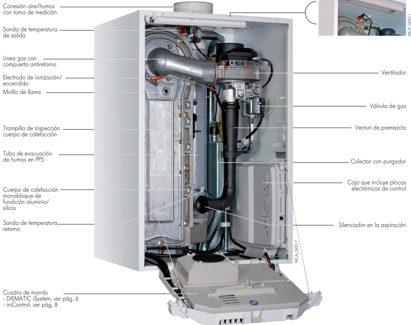
Detalles cuerpo de calefacción de fundición aluminio/silicio
