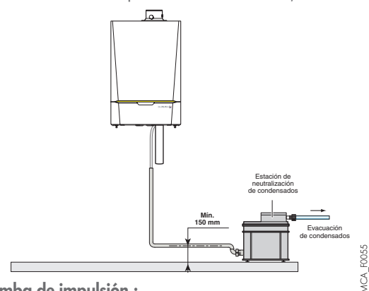
Estación de neutralización de condensados con bomba de impulsión :
