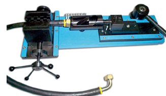
Introdutor rápido para racores Manual nipple inserter
