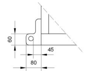
DETALLE PERNO DE SEGURIDAD
