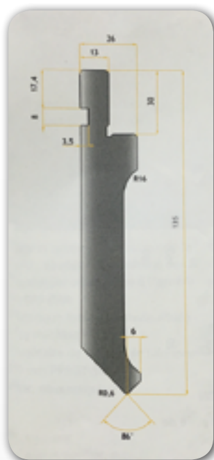
Punzón de altura 135mm
