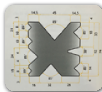
Bloque Multi-ue para plegadoras de 80 toneladas
