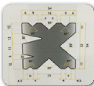
Bloque Multi-ue para plegadoras de 30 y 50 toneladas
