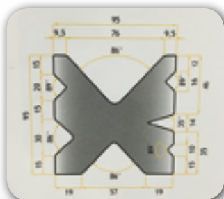
Bloque Multi-ue para plegadoras de 120 toneladas
