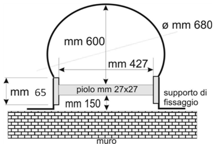
sezione scala con gabbia
