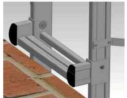
Plataforma de desembarco para reducir el espacio entre el último peldaño y la pared
