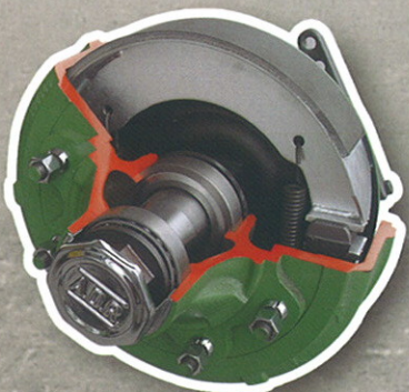
Eje agrícola con freno normal Agricultural axle with normal brake Essieu agricole avec frein standard
