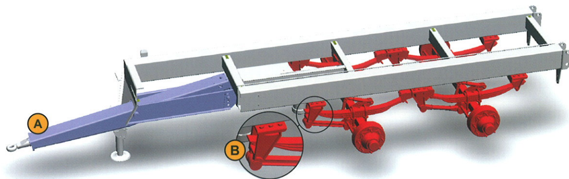
ESPARCIDOR CON TOLDO Y TAPA POSTERIOR CON MOLINETES SPREADER WITH A SHEET AND BACK COVER WITH BEATERS ÉPANDÉUR D'UNE FEUILLE ET LA FAÇADE ARRIÈRE AVEC GUINDEAUX
