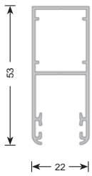
CÓD. 311650 Guía CR 53 x 22 10 x 6 m.
