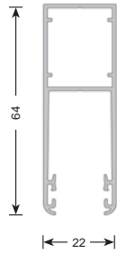
CÓD. 311651 Guía CR 64 x 22 8 x 6,5 m.
