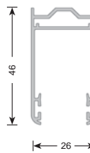
CÓD. 311655 Guía CT 46 x 26 10 x 6,5 m.
