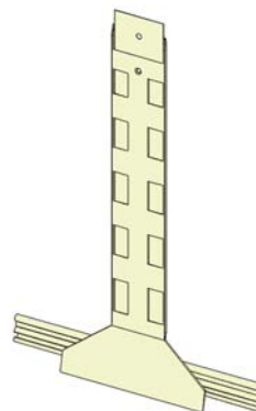
CÓD. 378223 Fleje tirante con taladros y funda protectora de plástico para la puerta VS-75R y VS-110
