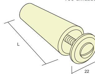
CÓD. 3754 41 L=40 mm. 42 L=60 mm. Tope con arandela 1.000 unidades
