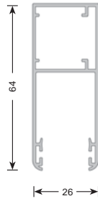
CÓD. 311652 Guía CR 64 x 26 8 x 6,5 m.
