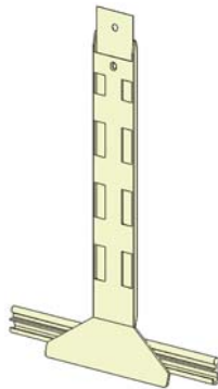
CÓD. 378227 Fleje tirante con taladros y funda protectora de plástico para la puerta VS-65
