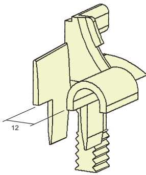
CÓD. 375450 Juego embudo nylon recto para guía de pvc y testero de aluminio
