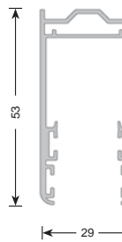
CÓD. 311656 Guía CT 60 x 29 10 x 6 m.
