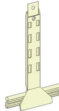
22_T para VS-41 CÓD. 3782 21_T para VS-45 Fleje tirante con taladros y funda protectora de plástico
