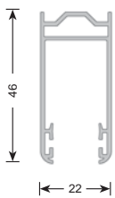
CÓD. 311654 Guía CT 46 x 22 10 x 6 m.
