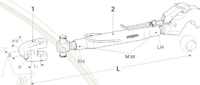
3° punto con husillo, cabezal y con articulación de horquilla y gancho
