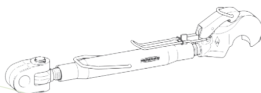
3º punto con husillo, cabezal y con articulación de horquilla y gancho
