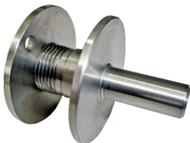
328M Punto de giro techillo para 301M Top pivot pin for 301M
