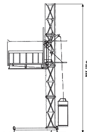
CESTA DE PLADUR / PLASTERBOARD BASKET
