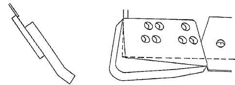
FORJADAS EMBUTIDAS 3G, 1U, 7T
