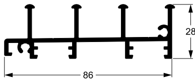
Marco inferior para 3 carriles
