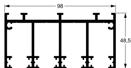
Marco superior de 4 carriles
