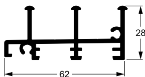
Marco inferior para 2 carriles
