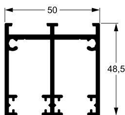
Marco superior de 2 carriles
