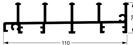
Marco inferior para 4 carriles
