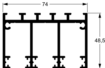
Marco superior de 3 carriles
