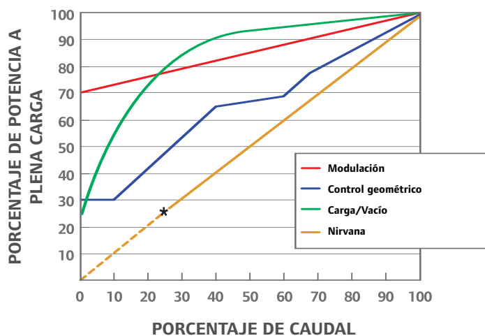
Comparación de los controles de capacidad en compresores rotativos
