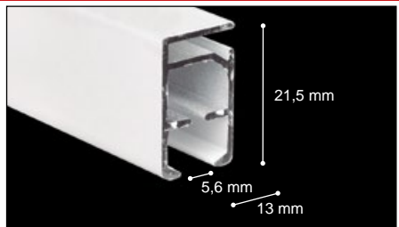
Perfil de aluminio blanco
