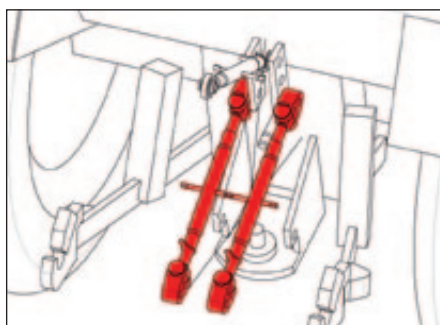
Kit de estabilizadores por cardanes
