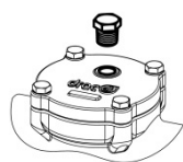
Conexión de venteo (sólo tapa atornillada)
