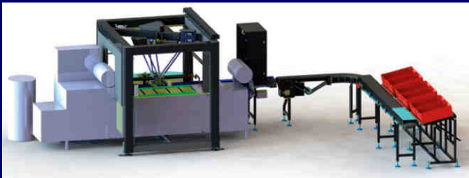
ROBOT TRÍPODE DELTA CALIBRA
