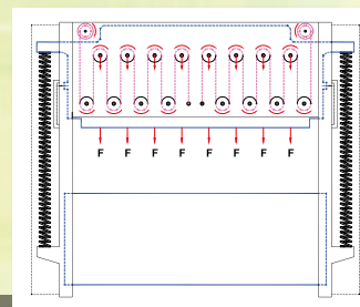
Distribución de fuerzas constante
