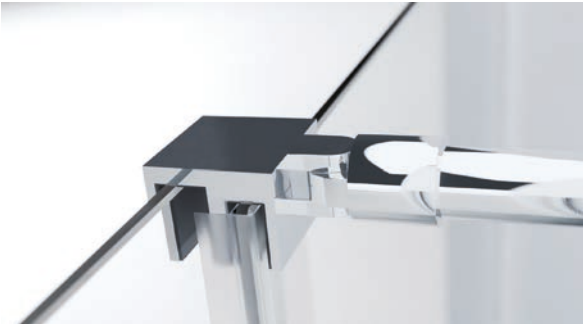
Pinza guía superior.
