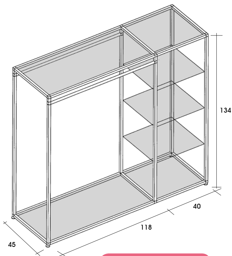
ref. 3846 20x20 ref. 3946 25x25 ESTANTERÍA + 2 BARRAS PENDERIE
