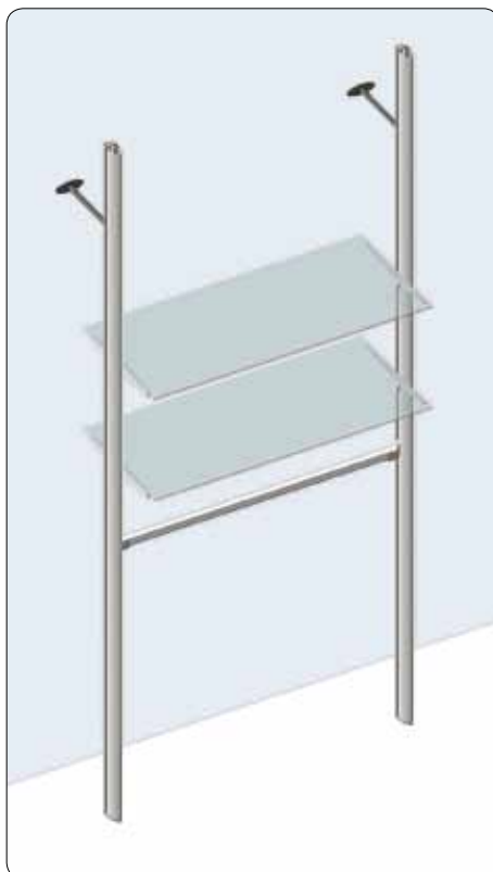
FIJACIÓN A PARED MEDIANTE EL BRAZO TELESCÓPICO 4545
