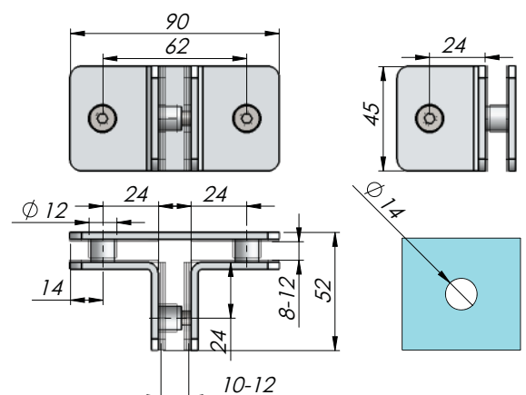
4099/022 Herraje fijo pared-vidrio 90° Inox brillo
