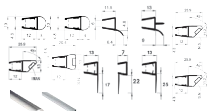
TAPAJUNTAS - BURLETES 116
