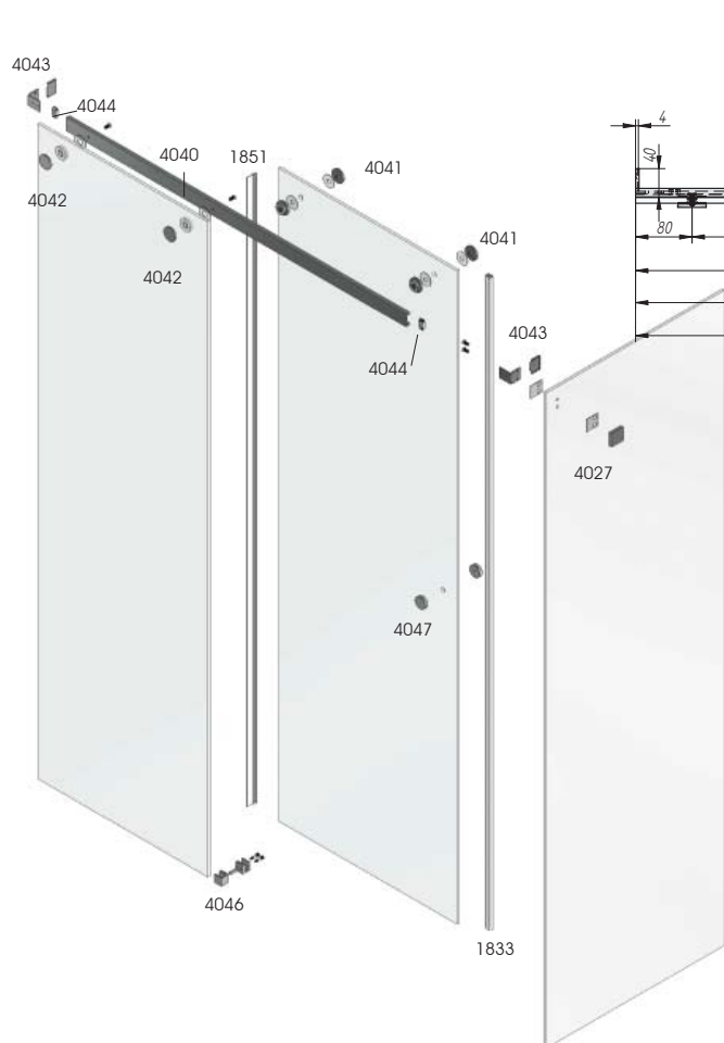
90° 1 PUERTA
