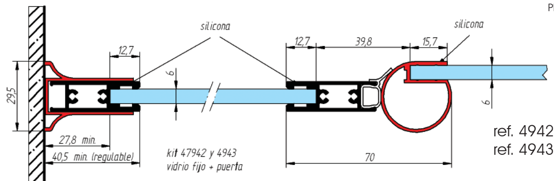
PERFIL INTERMEDIO REGULABLE
