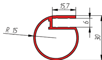
PERFIL BISAGRA
