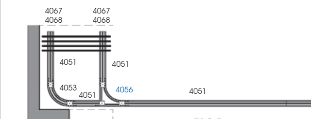
TIPO E. ALMACÉN A LA IZQUIERDA 4051/101 perfil de aluminio 4056/001 esquina 90° izq. 4053/001 curva 90° 4067/001 stop carril superior (2 u.) 4068/001 tapa final carril (2 u.)
