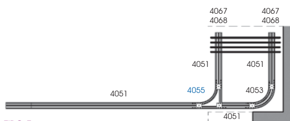
TIPO F. ALMACÉN A LA DERECHA 4051/101 perfil de aluminio 4055/001 esquina 90° der. 4053/001 curva 90° 4067/001 stop carril superior (2 u.) 4068/001 tapa final carril (2 u.)
