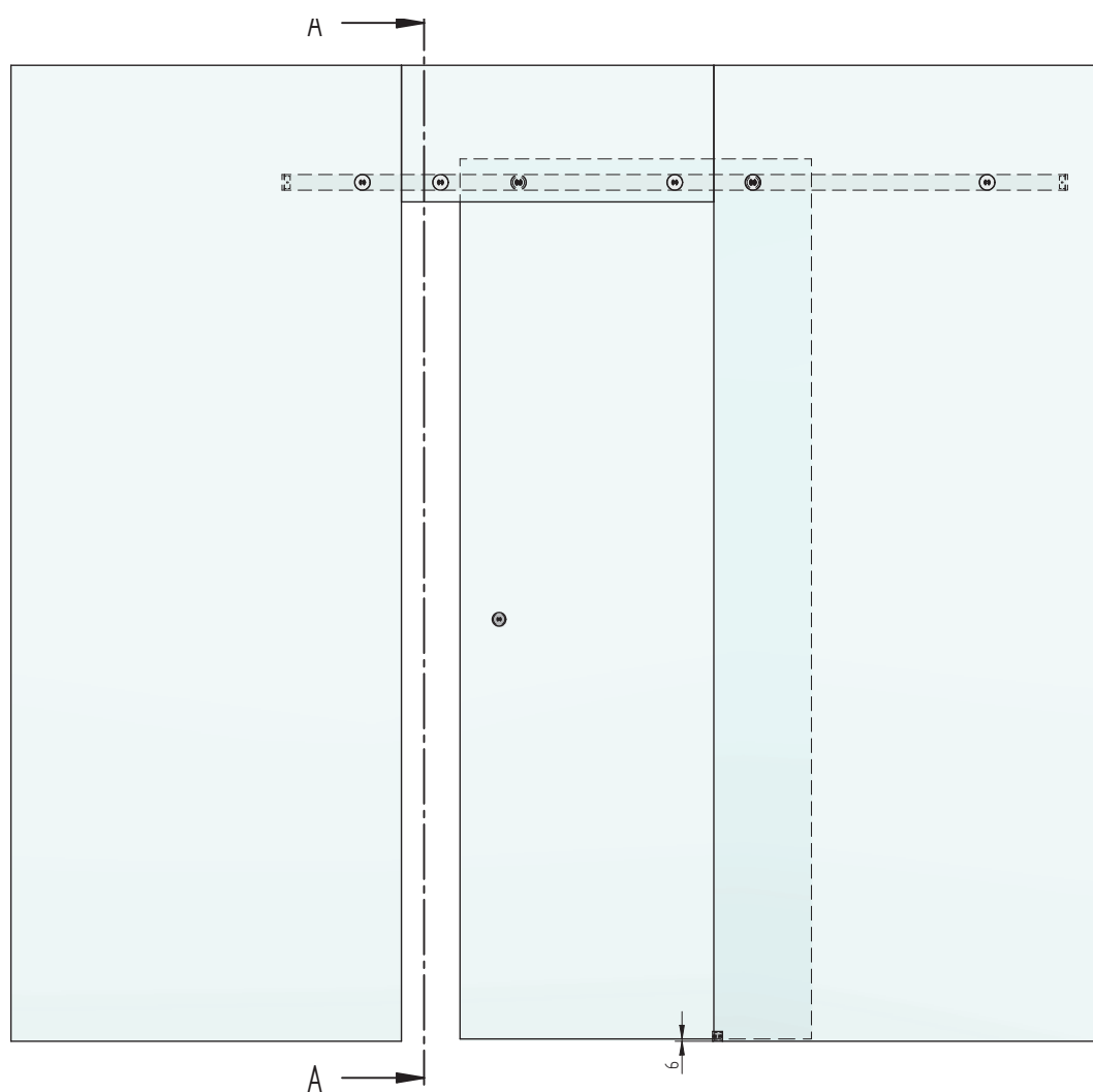
CORTE A-A
