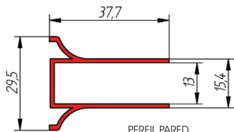
PERFIL PARED
