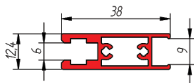
PERFIL INTERMEDIO REGULABLE
