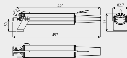
04791020 ST450 carrera 180 - para ventanas PROYECTANTES
