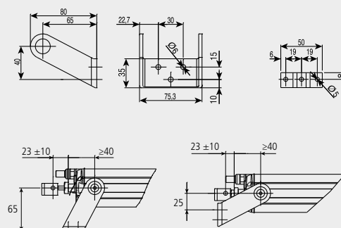
04792020 ST450 carrera 300 - para ventanas PROYECTANTES
