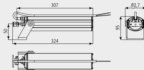
04791020 ST450 carrera 180 - para ventanas PROYECTANTES
