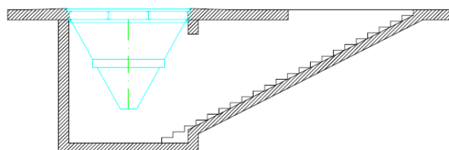
UN SENO SALIDA LIBRE - REJA DE PASO FIJA
