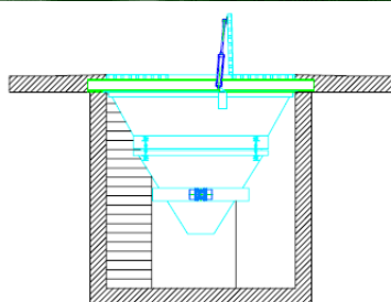
CONO VIBRANTE - REJA DE PASO ABATIBLE
