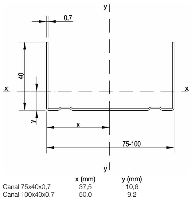
Figura 2.2: Canal tipo.
