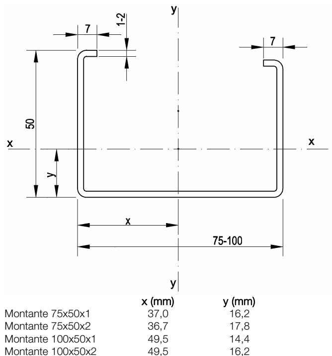
Figura 2.1: Montante tipo.
