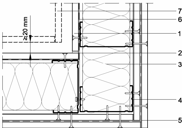
Figura 6.6: Esquina saliente del sistema Aquapanel® Outdoor W384.
