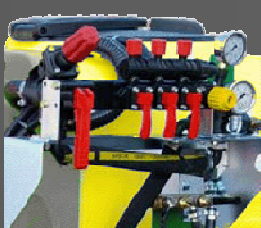
DISTRIBUIDOR MANUAL O ELECTRICO DE 3 O 5 VIAS
