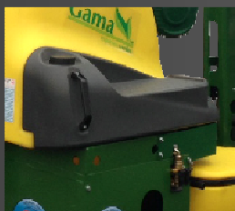
DEPOSITO AUX. LAVAMANOS INTEGRADO EN ESCALERA DE ACCESO A TAPADERA
